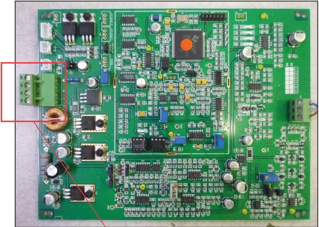
Разъёмы питания
